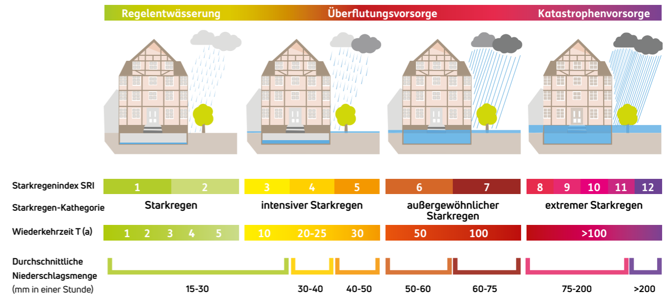
Abbildung 8: Starkregenindex mit Wiederkehrzeiten und Starkregenkategorien. (nach Schmitt et al.)
