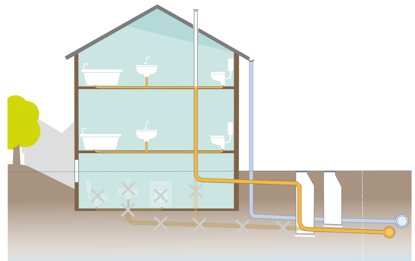
Abbildung 19: Rückbau von Entwässerungsgegenständen im Keller
