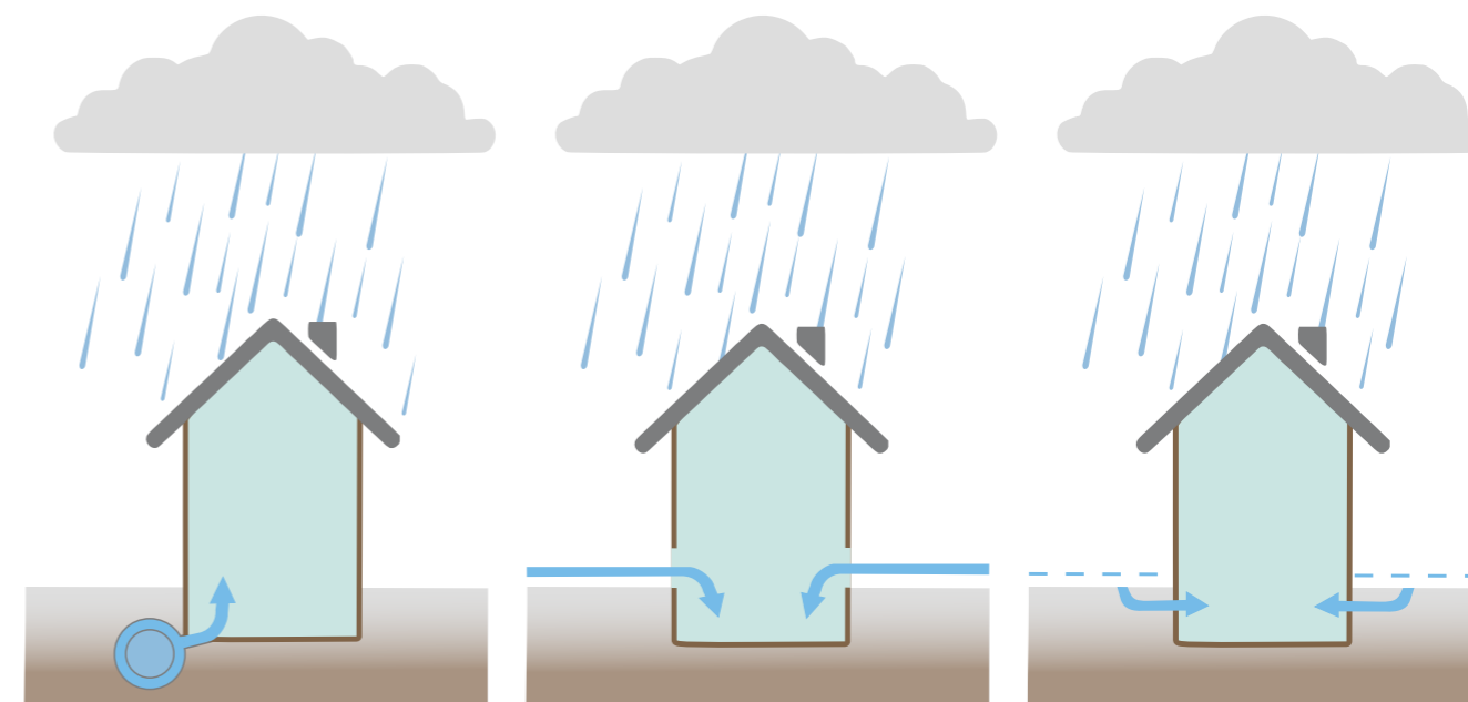
Abbildung 11: Wege, wie Wasser ins Gebäude gelangen kann
